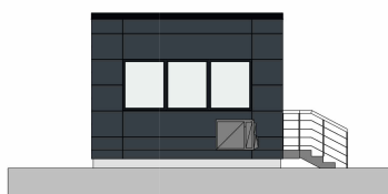
Syd_facade 1 : 100
